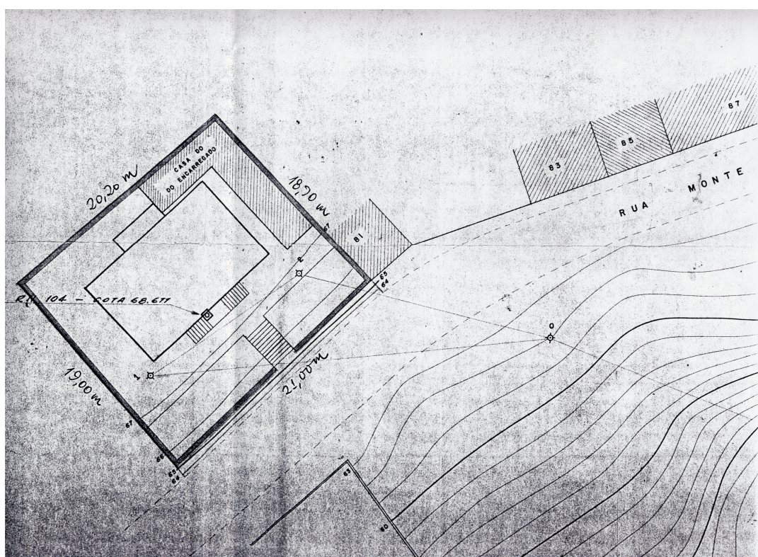
Planta de situação. Fonte: GB - SURSAN
